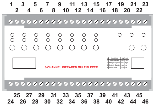
Abb. 1: Klemmen-Nummerierung
