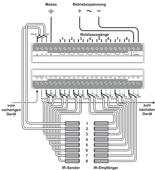
Abb. 2: Anschlussschema
