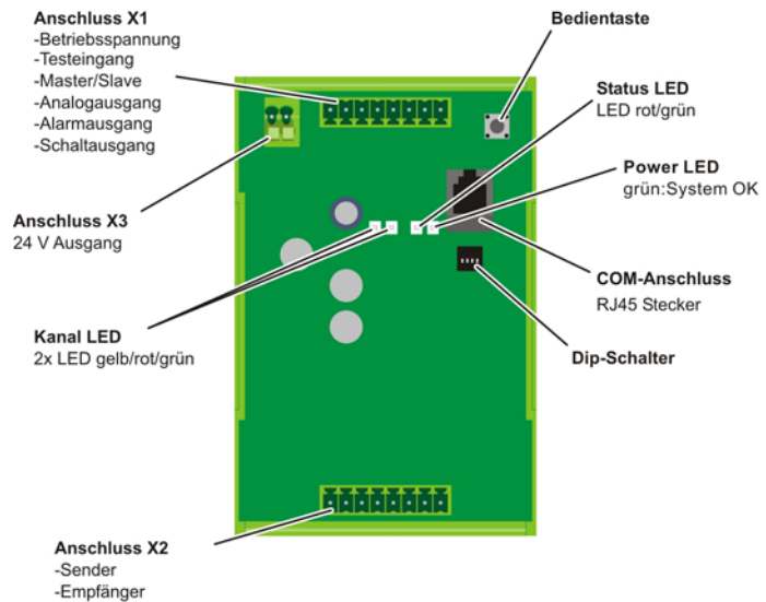
Bedienelemente ICL-2000
