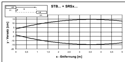
Bild 4: Leistungsdiagramm STB... / SRSx...
